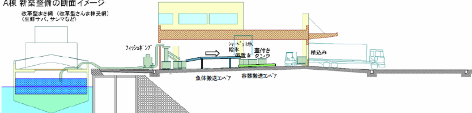
A棟 新築整備の断面イメージ
